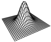
Distribución normal multivariada
