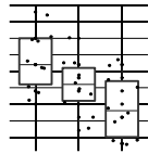
Pruebas de hipótesis multivariadas
