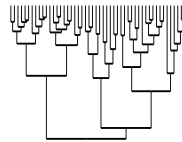
Análisis de conglomerados
