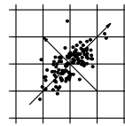
Análisis de componentes principales
